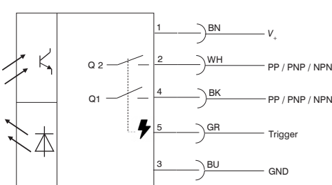
CLS1000-2Q-xx-T
