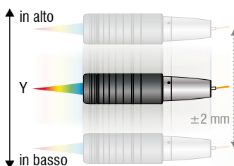
❷ Max. spostamento in Y \pm 2 mm
