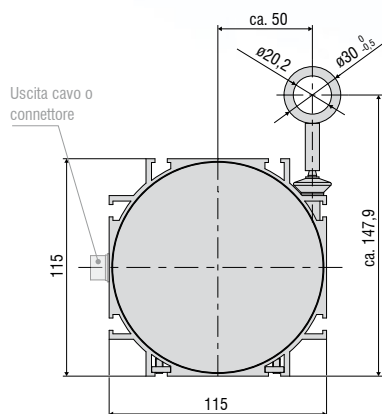
Uscita HTL/TTL
