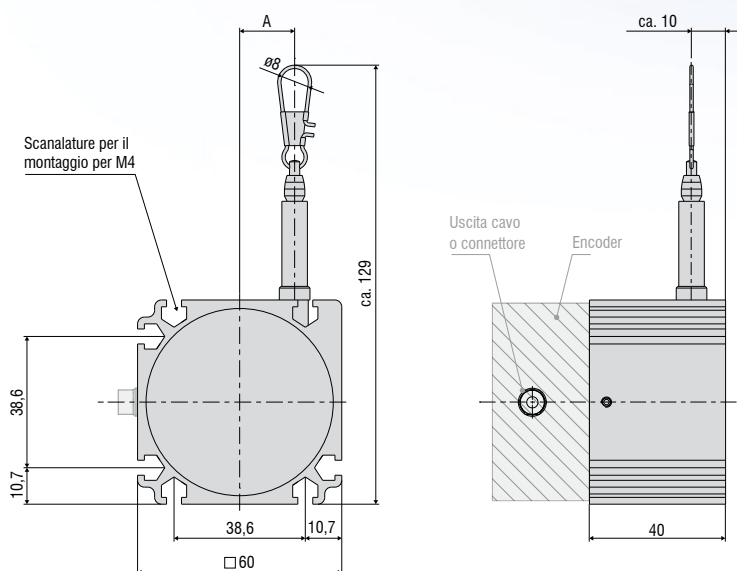
Uscita HTL/TTL
