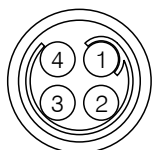
Vista lato da saldare, connettore femmina 4 poli
