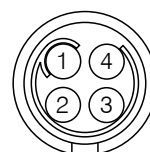
Vista lato da saldare, spina del cavo a 4 poli
