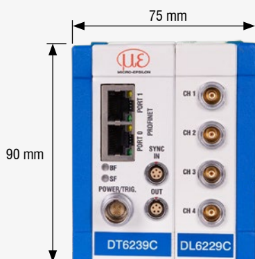
DT6229 con 2 o 4 canali di misurazione
