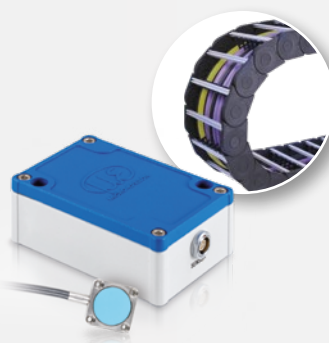
Sensori attivi per catene portacavi e lunghi percorsi capa NCDT 6114
