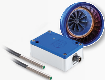
Misurazione del numero di giri capaNCDT CST6110
