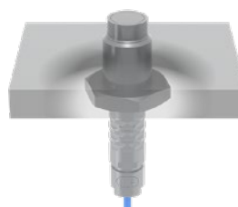
Bloccato sul retro mediante dado
